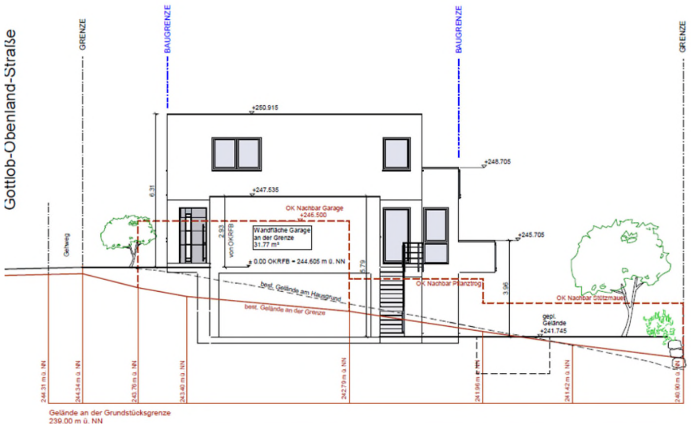
Ansicht West
