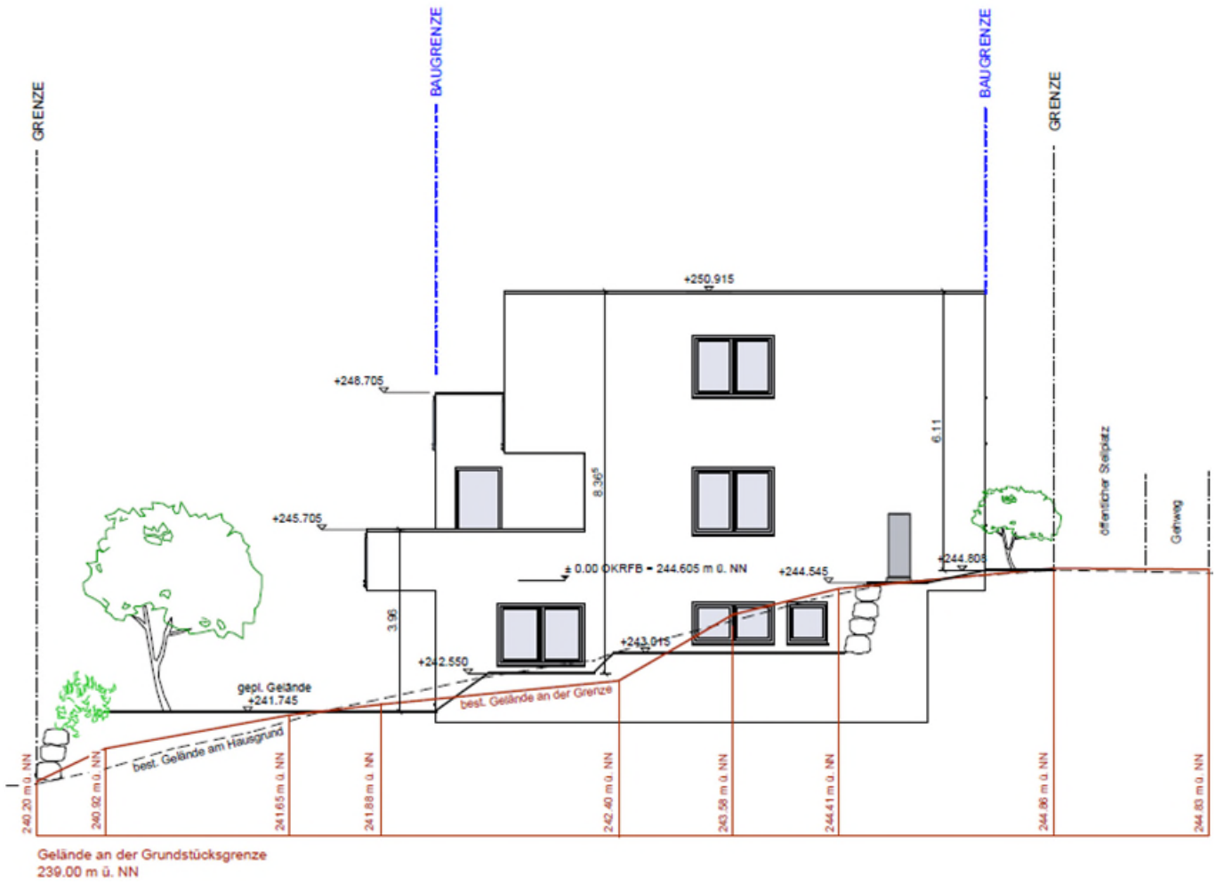
Ansicht Ost
